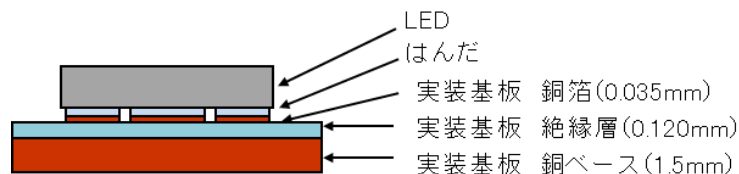
図4 実装構造
