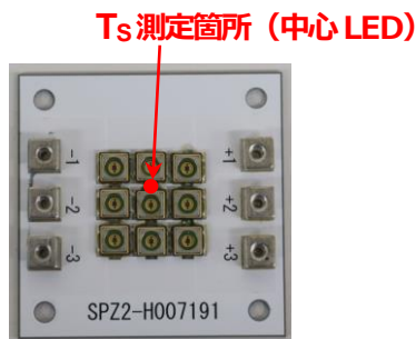
写真4 実装状態
