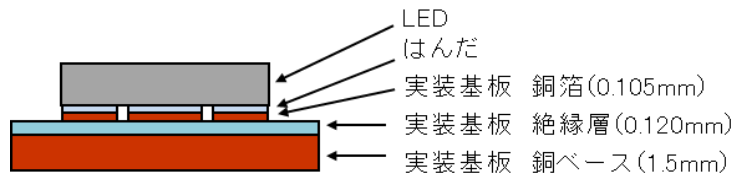
図3 実装構造
