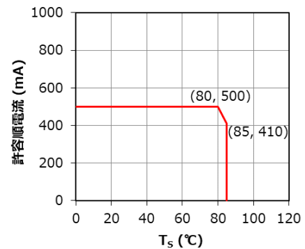
図1 T_S - 許容順電流特性
