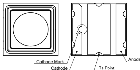
図2 T_S 測定ポイント
