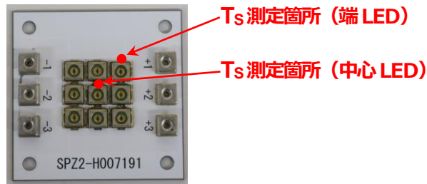
写真 10 LED を 9 個搭載した LOB の T_s 測定位置
